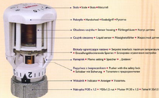
Głowica termostaticzna typ GZ.03
